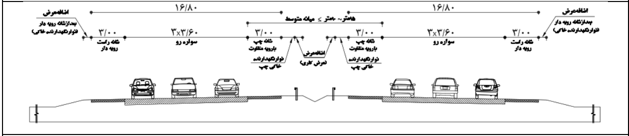
F۱۱- آزادراه شش خطه با DDHV کمتر از ۲۵۰ با میانۀ متوسط
