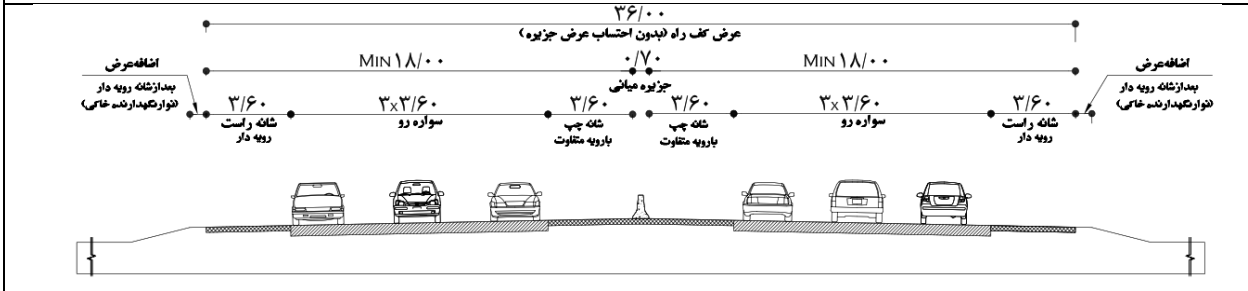
F۴- آزادراه شش خطه با DDHV برابر و بیشتر از ۲۵۰
