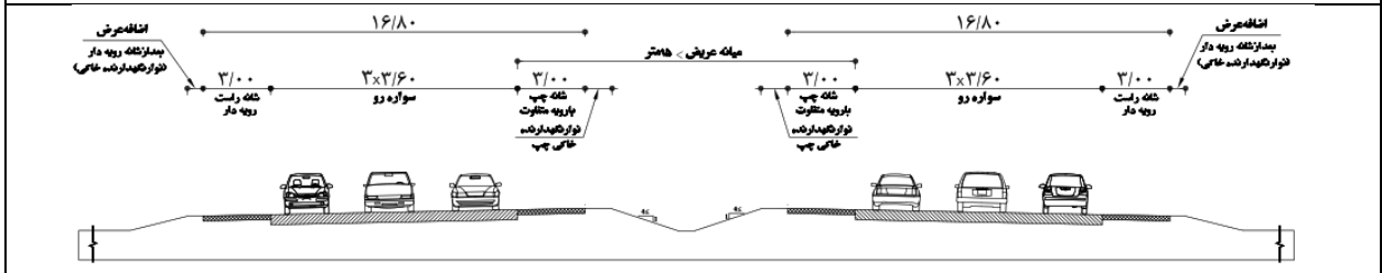
F۱۲- آزادراه شش خطه با DDHV کمتر از ۲۵۰ با میانۀ عریض
