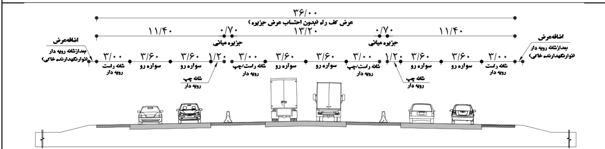
F۵- آزادراه با سه کف راه با DDHV کمتر از ۲۵۰
