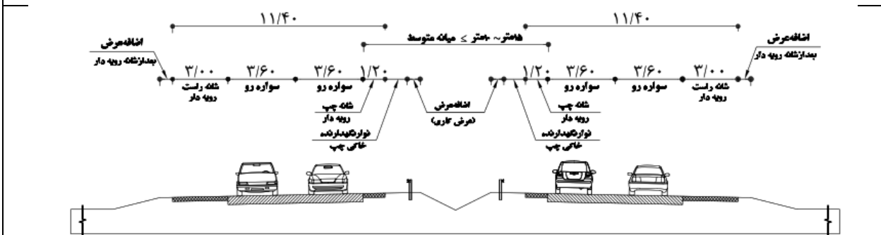
F۷- آزادراه چهار خطه با DDHV کمتر از ۲۵۰ با میانه متوسط
