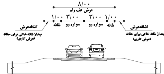
L۳- راه محلی دو خطه با ADT بین ۲۰۰۰ تا ۶۰۰
