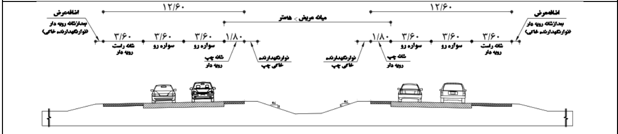
F۱۰- آزادراه چهار خطه با DDHV برابر و بیشتر از ۲۵۰ با میانۀ عریض
