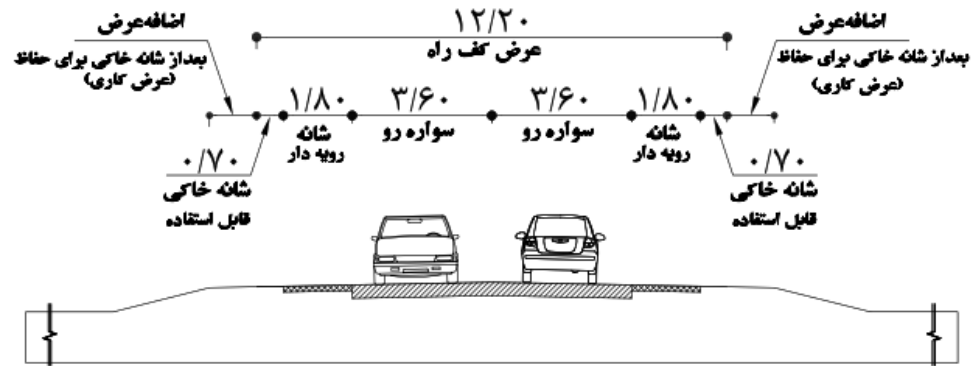
A۴- راه شریانی دو خطه با ADT بیشتر از ۲۵۰
