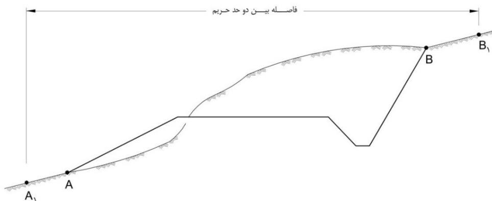
شکل ۶-۱۸- حریم راه
