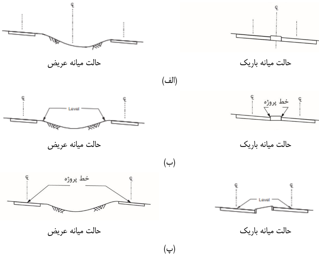
شکل ۵-۳- دوران بریلندی حول لبه خارجی در سواره روی با شیب عرضی یک طرفه
