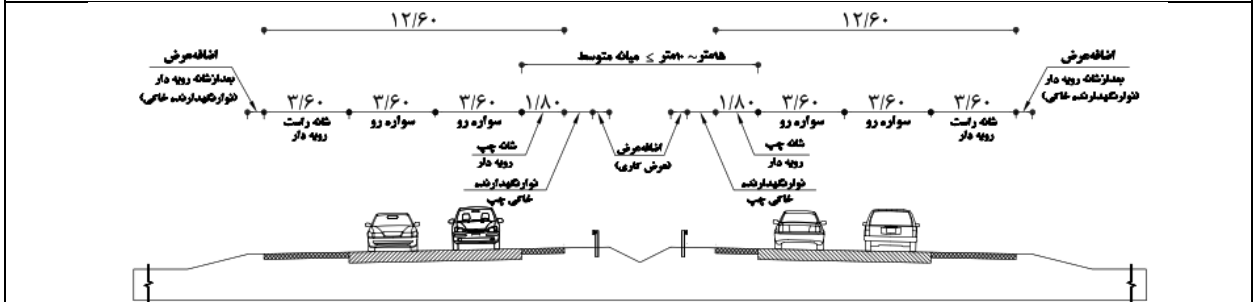
F۹- آزادراه چهار خطه با DDHV برابر و بیشتر از ۲۵۰ با میانۀ متوسط
