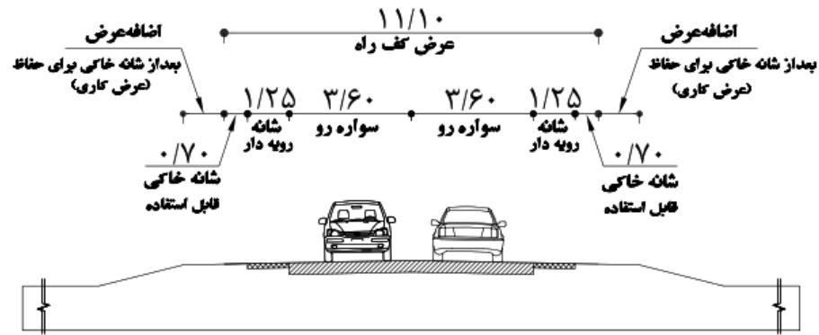
A۳- راه شریانی دو خطه با ADT کمتر و برابر ۲۵۰
