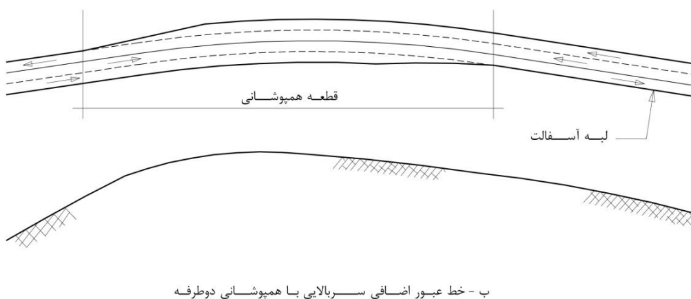
شکل ۵-۱۴ - خط‌های کمکی سربالایی در راه‌های دو خطه دو طرفه
