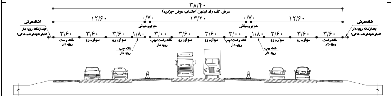
F۶- آزادراه با سه کف راه با DDHV برابر و بیشتر از ۲۵۰
